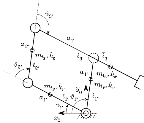
Fig. 7.12. Parallelogram arm
