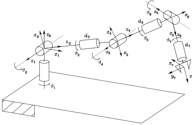
Fig. 2.27. DLR manipulator
